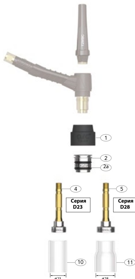
КВАРЦЕВЫЕ СОПЛА
