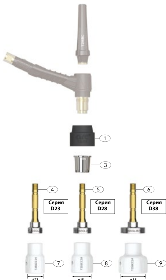
КЕРАМИЧЕСКИЕ СОПЛА
