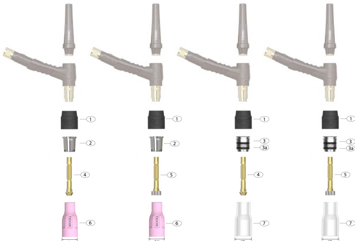
СЕРИЯ СО СТАНДАРТНОЙ ЦАНГОЙ И КЕРАМИЧЕСКИМ СОПЛОМ
