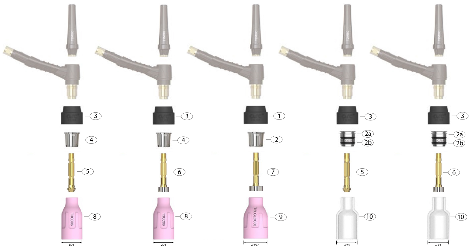
СЕРИЯ СО СТАНДАРТНОЙ ЦАНГОЙ И КЕРАМИЧЕСКИМ СОПЛОМ
